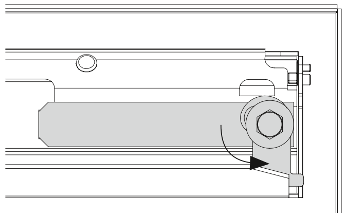
Klappenverschluss gesperrt
