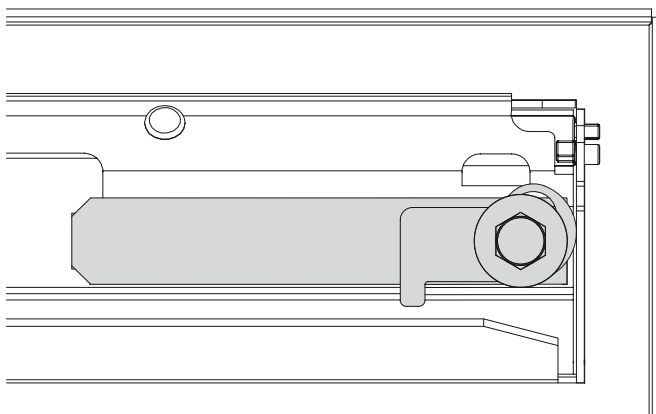
Klappenverschluss im Normalbetrieb
